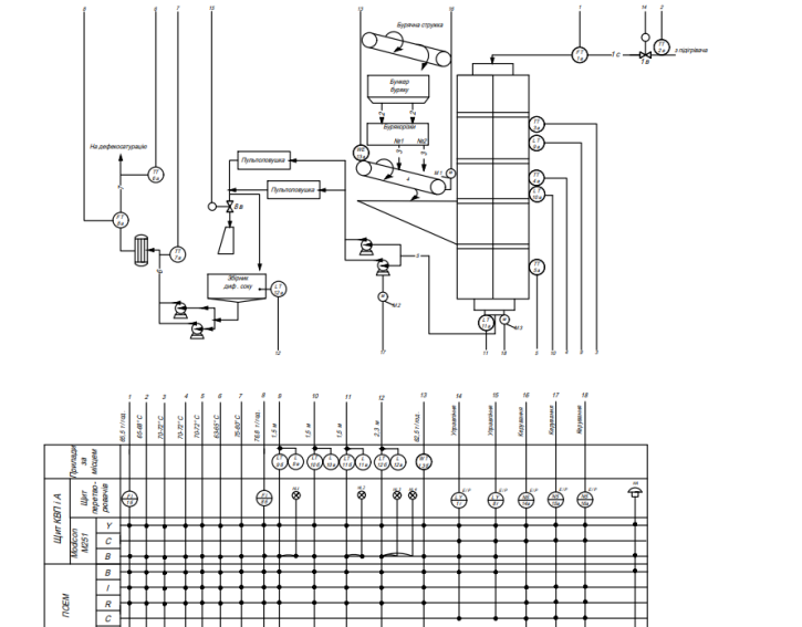
Рисунок 1 – Функціональна схема автоматизації дифузійного апарату колонного типу
